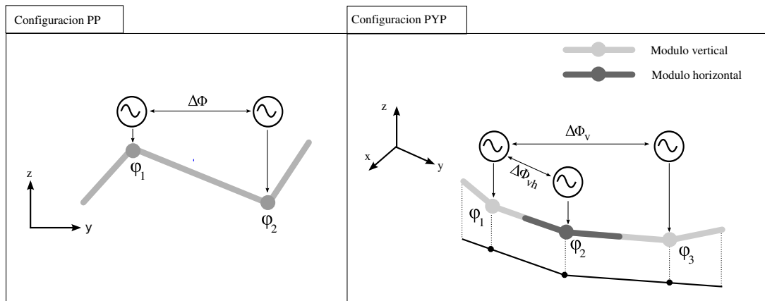
Figura 6.6: Modelo de control de las configuraciones mínimas PP y PYP
