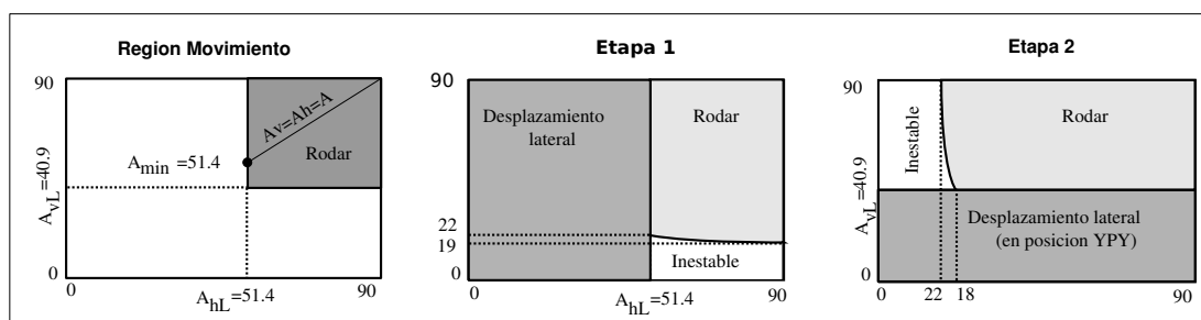
Figura 6.31: Regiones de movimiento para el caso de estudio: Etapa 1, 2 y la total
